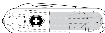
Frente translúcida con LED, emblema siempre en el frente, longitud 58 mm
